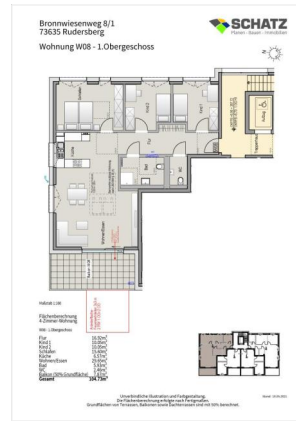
Grundriss W08
