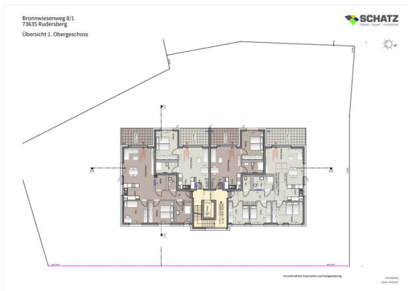
10 Grundriss 1. OG
