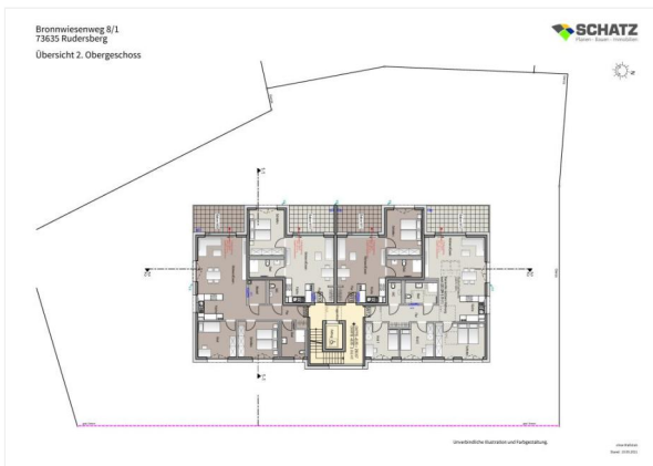
11 Grundriss 2. OG
